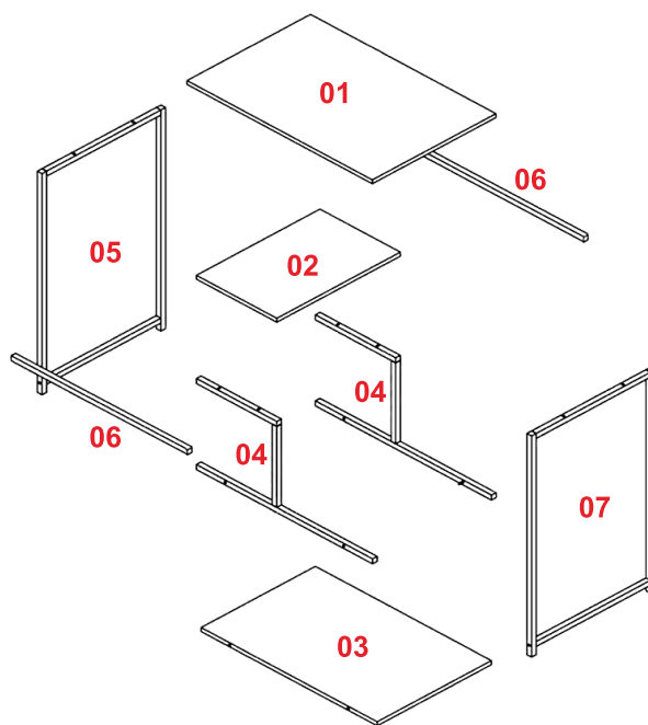
Produto Desmontado
